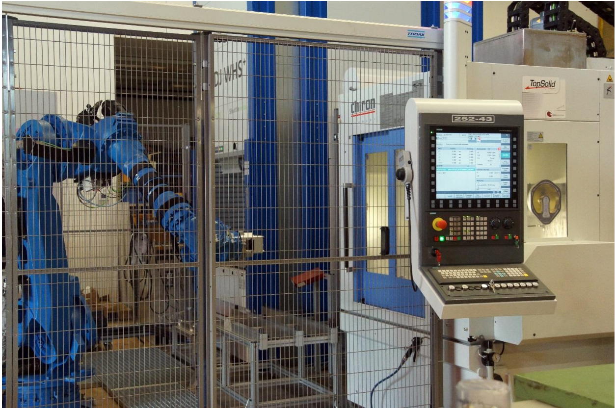
Foto 5: Fertigungszelle mit Chiron Fräscnter und 6-Achsen Knickarm-Roboter
